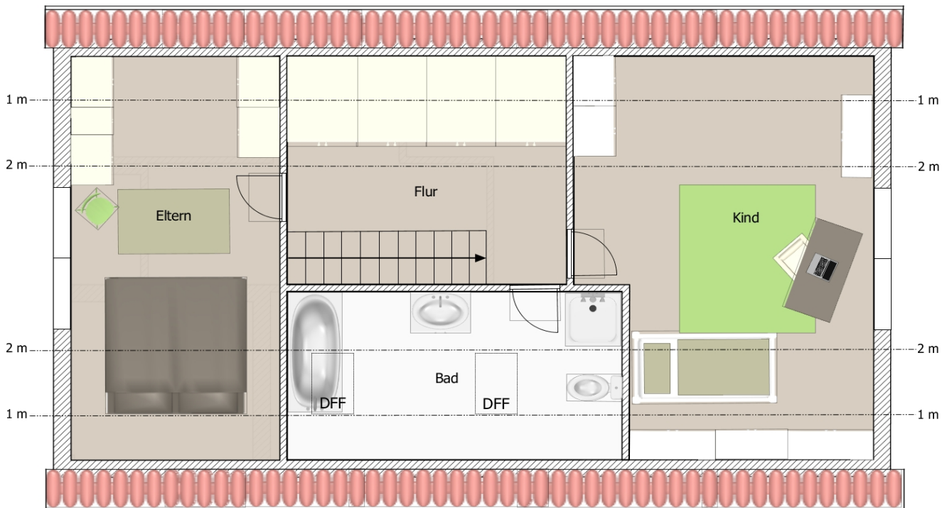
Grundriss DG
